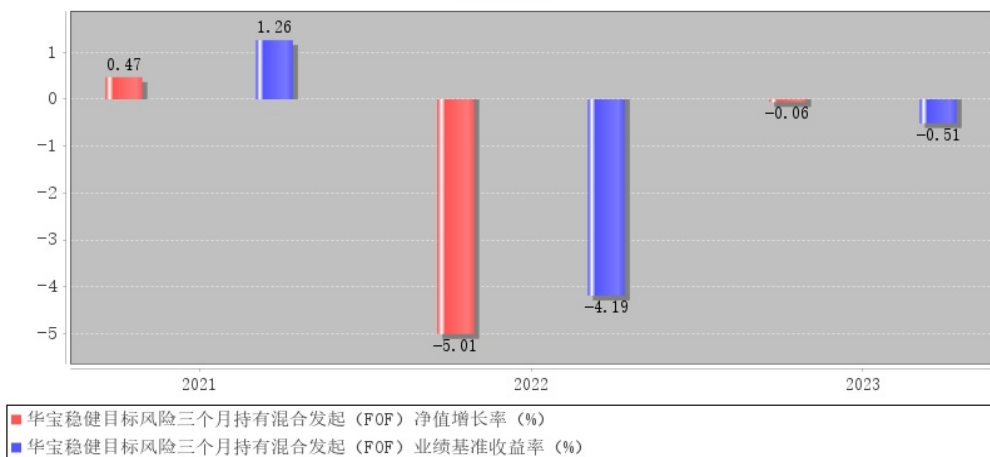
华宝稳健目标风险三个月持有混合发起（FOF）每年净值增长率与同期业绩比较基准收益率的对比图
